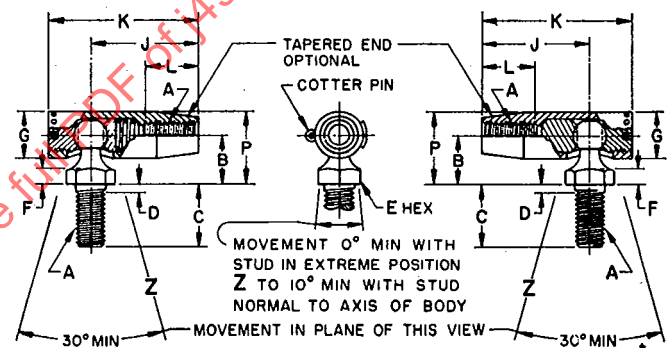
FIG. 3—TYPE B
