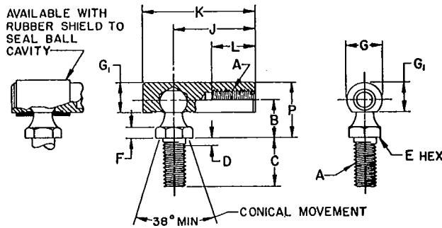
FIG. 8A—STYLE 1
