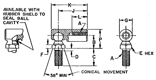
FIG. 8B—STYLE 2
