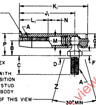
FIG. 2—TYPE AL
