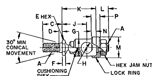
FIG. 7B—STYLE 2
