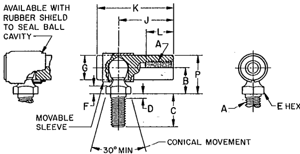
FIG. 8C—STYLE 3 b
