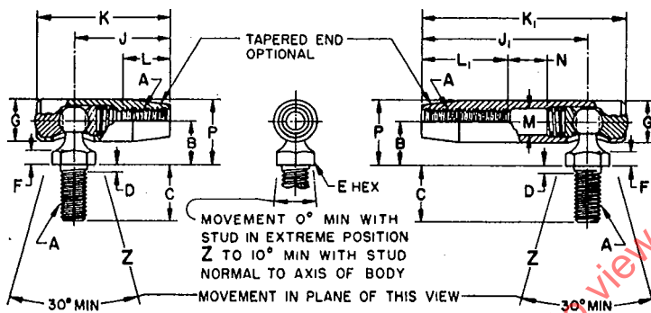
FIG. 1—TYPE A
