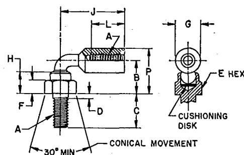
FIG. 5—TYPE D*
