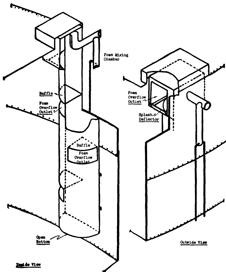
Fig. A-302 (b) (3). Foam Chute.
