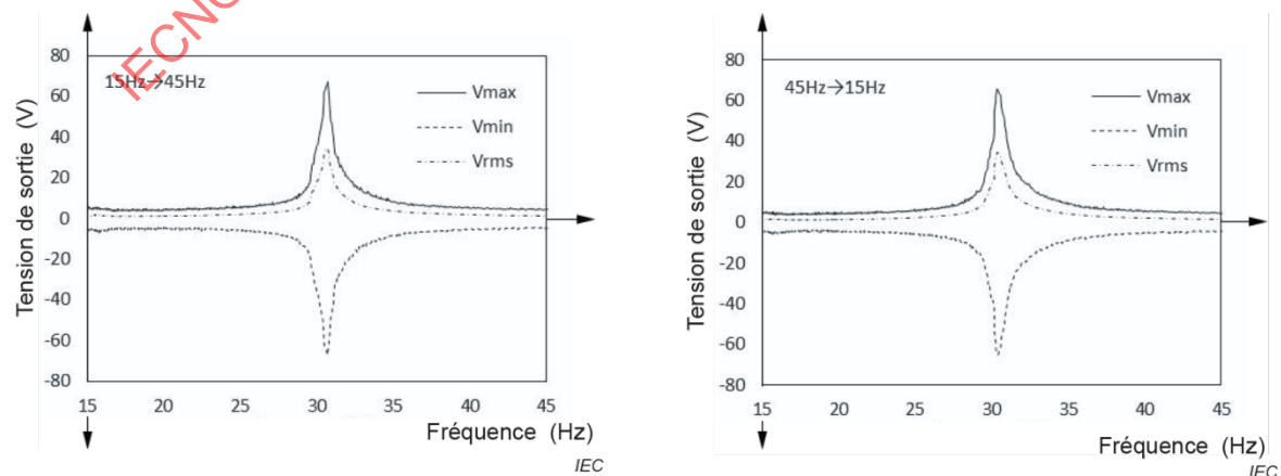
c) 0,98 m/s 2 pour le balayage ascendant
