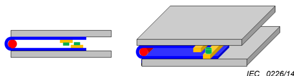
Figure 2 – Appareillage d'essai de flexion statique
