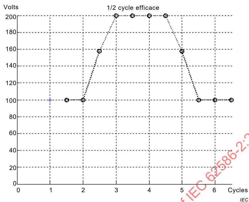
Figure 8 – Détail 2 de la forme d'onde pour les essais des surtensions conformément à l'essai A4.1.2
