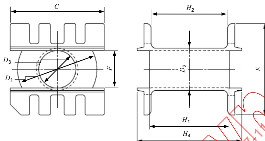
Figure A.2 – Dimensions principales des carcasses pour les noyaux EC90
