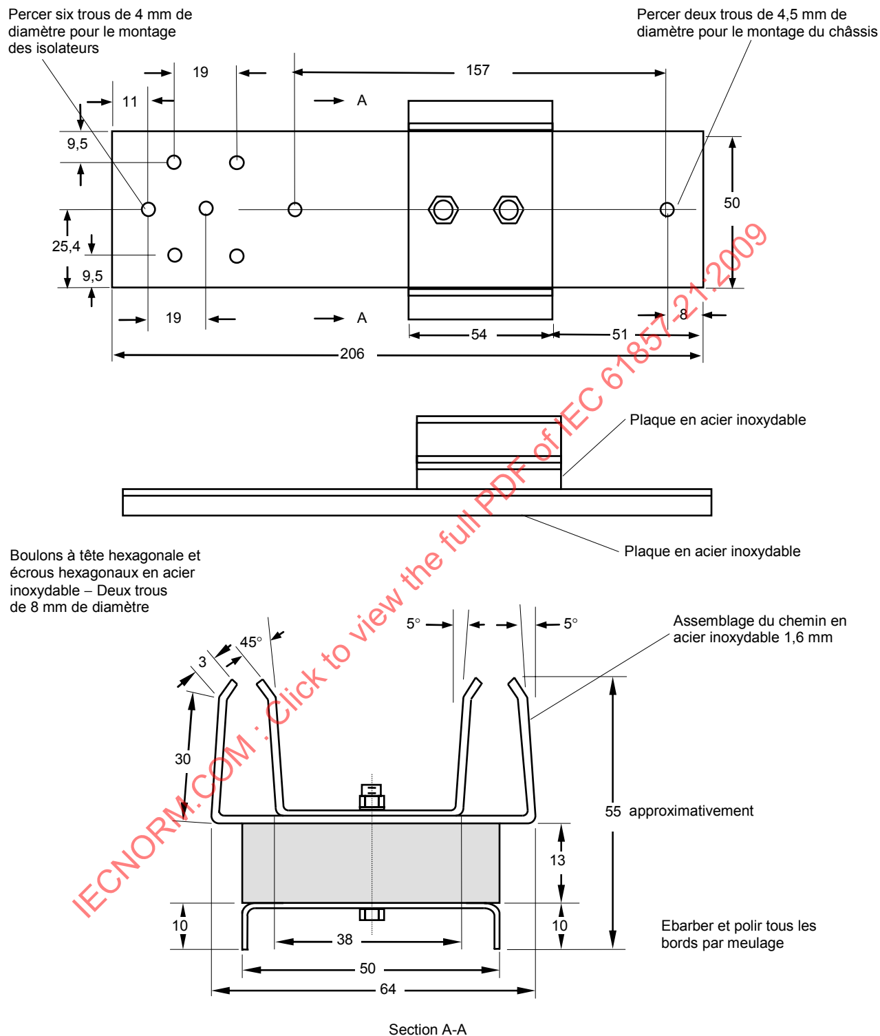
Figure 3 – Schéma de fabrication d'un châssis de GPM-TC
