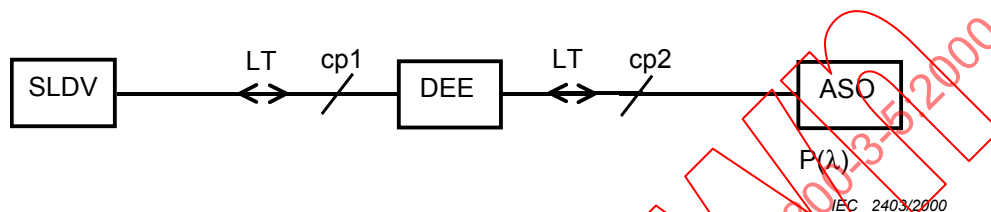
Figure 3 – Méthode à l'aide d'un analyseur de spectre optique – Etape 1
