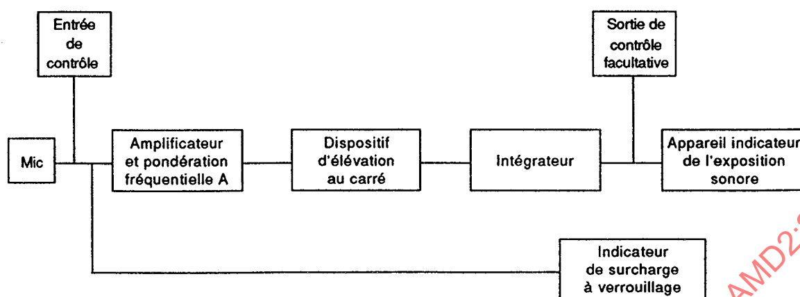
Figure 1 – Eléments fonctionnels d'un exposimètre acoustique individuel
