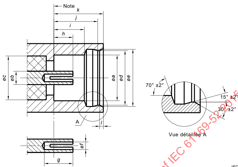
Figure 2 – Connecteur avec contact central femelle
