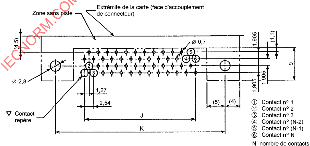
Figure 15b – Connecteur pour 14, 26, 50 et 110 contacts (verrouillage à vis)
