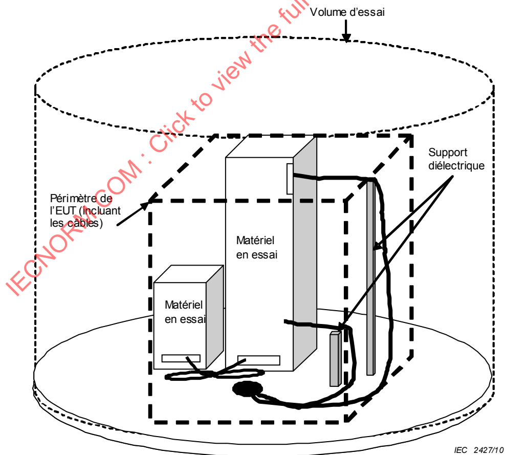
Figure 8 – Exemple de montage d'essai pour un matériel posé au sol
