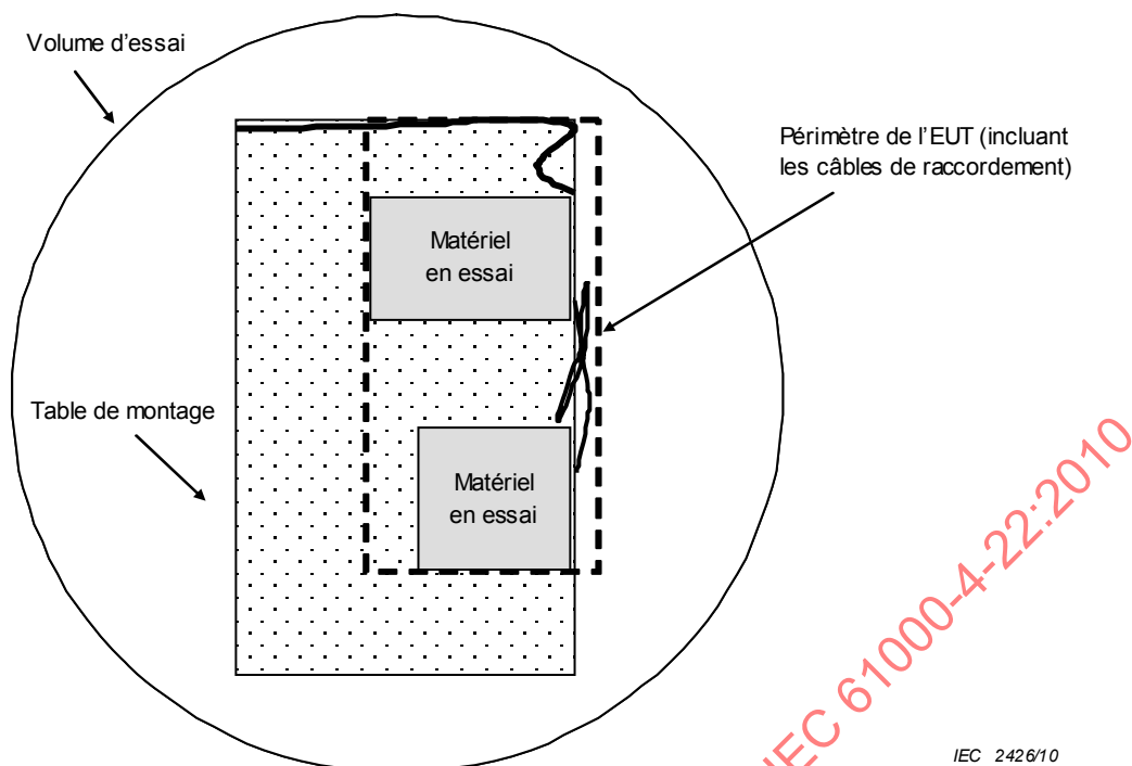
Figure 7 – Exemple de montage d'essai pour un matériel posé sur table, vue de dessus
