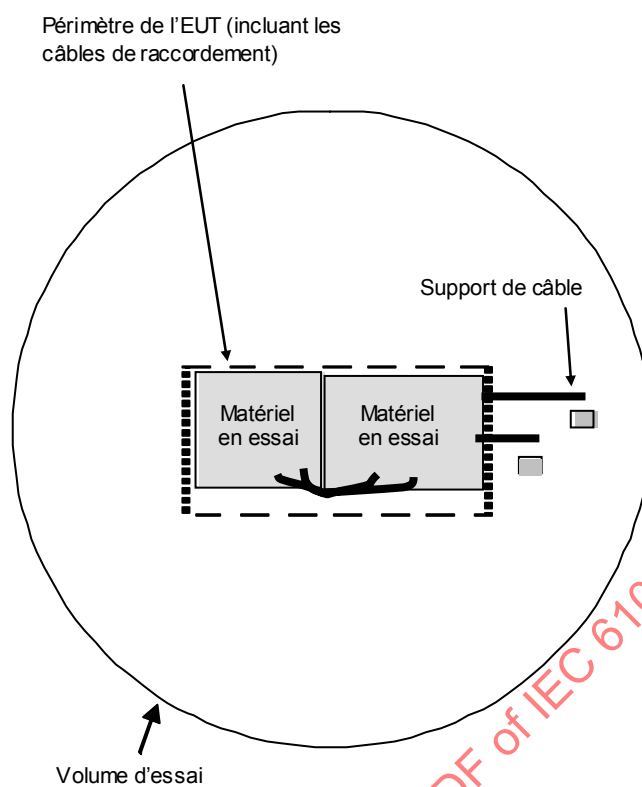
Figure 9 – Exemple de montage d'essai pour un matériel posé au sol, vue de dessus
