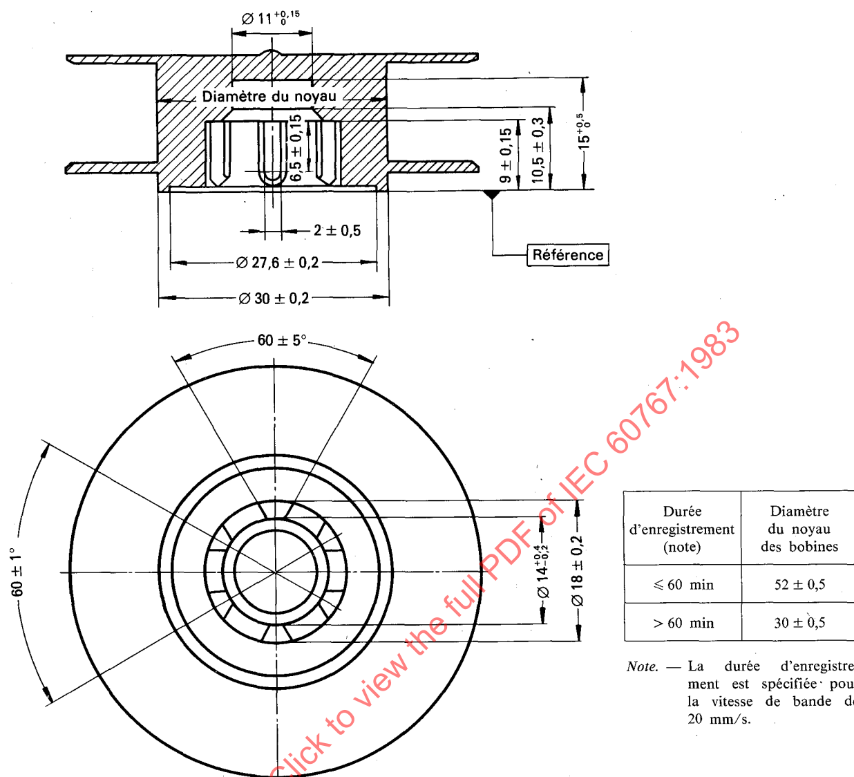
FIG. 6. — Bobine de cassette.
