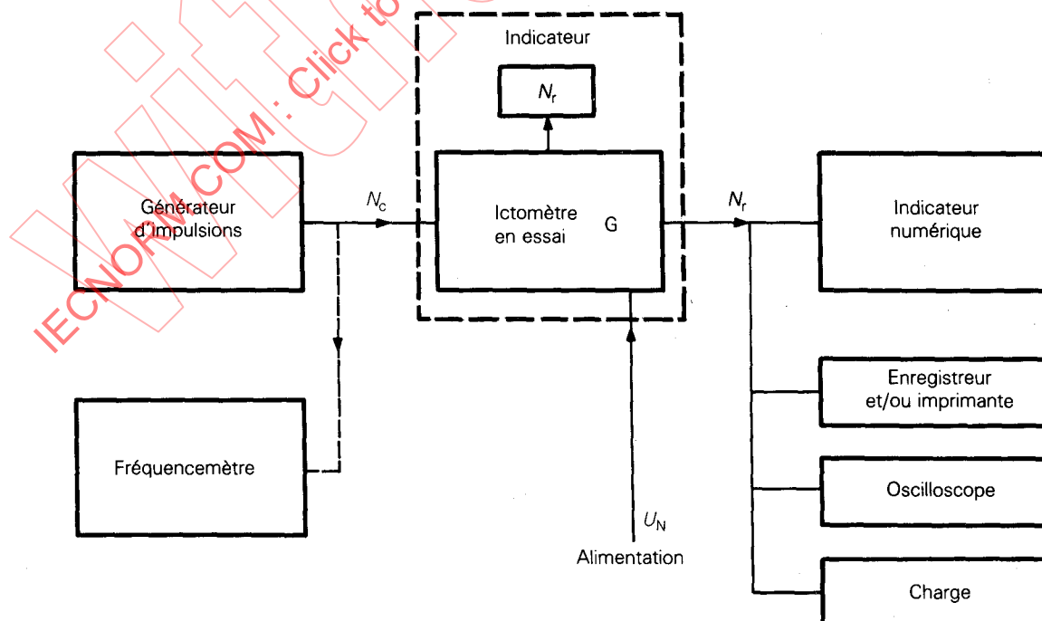
FIG. 2. — Disposition générale pour les essais.
