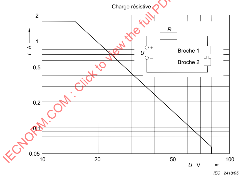
Figure 35 – Courant maximal admissible I en fonction de la tension maximale admissible U mesuré dans un circuit purement résistif dans un ENVIRONNEMENT RICHE EN OXYGÈNE (voir 11.2.2.1)
