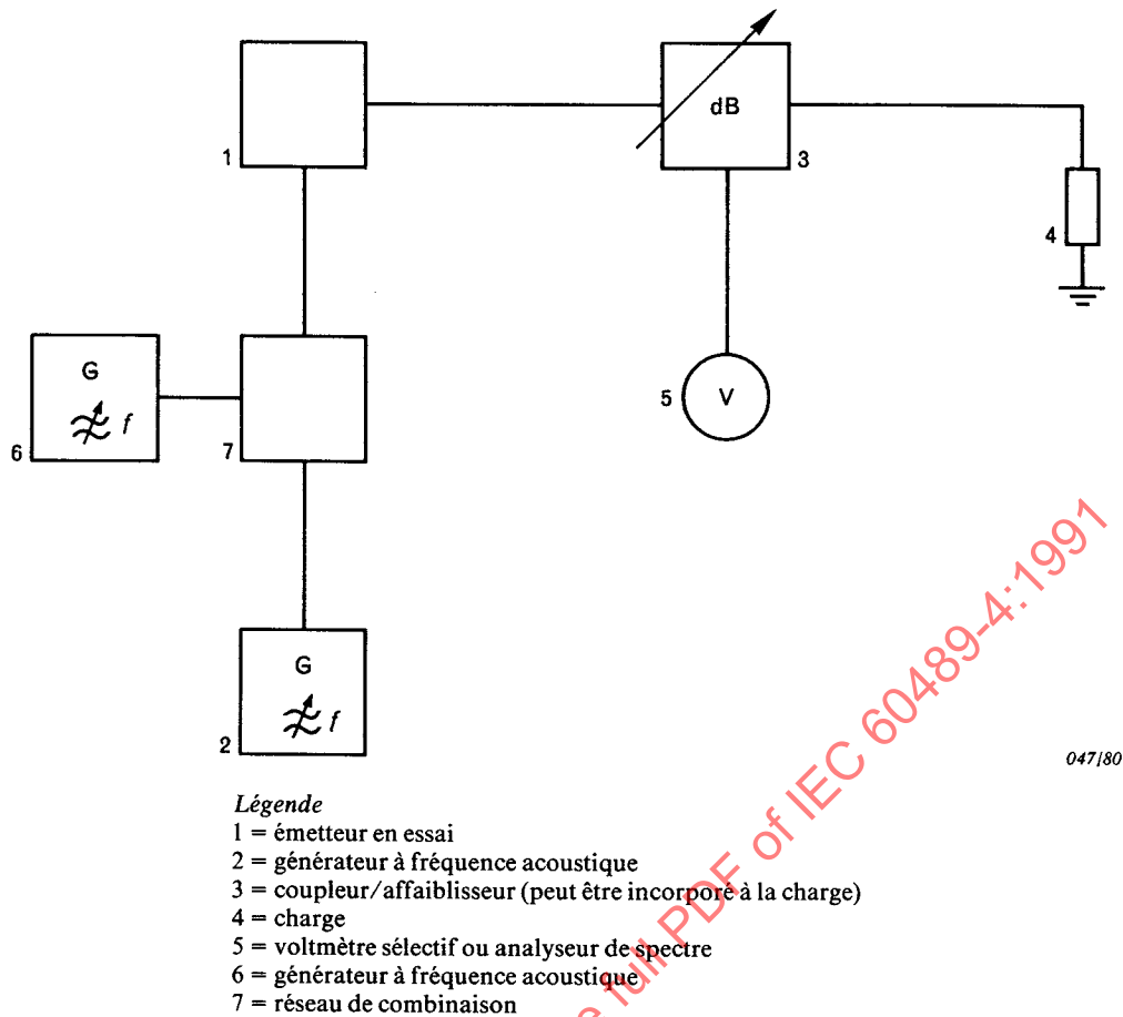
FIG. 9. — Montage de mesure des caractéristiques de l'émetteur.
