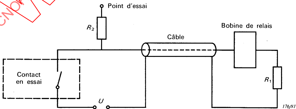
FIG. 5. — Charge en courant continu par câble et relais combinées. R_1 : voir paragraphe 4.1. R_2 \geq 50 \text{ k}\Omega .
