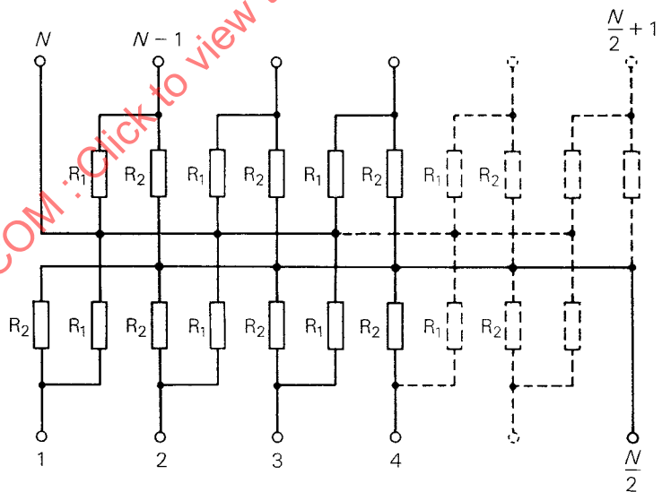
SCHÉMA DIAGRAM J
